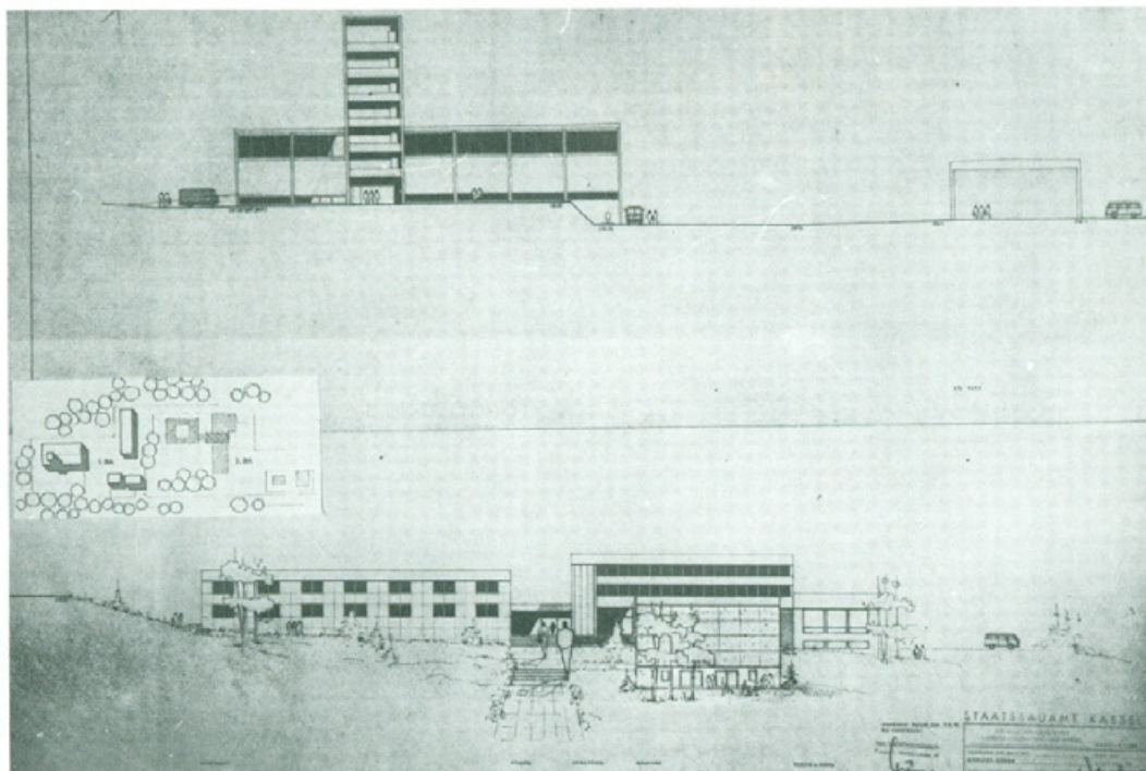
Bauzeichnung für den Neubau oben Übungshalle mit Übungsturm unten Unterkünfte- und Verwaltungsgebäude
