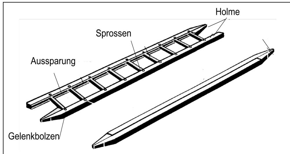
Abb. 16: Klappleiter
