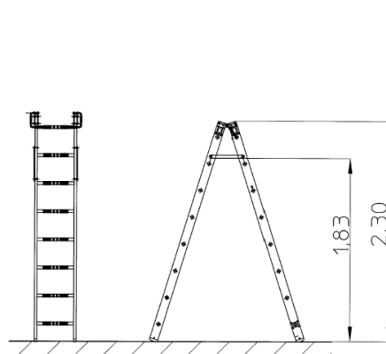
Abb. 25: Stehleiter
