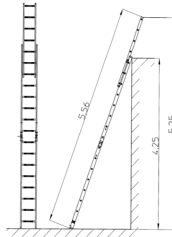
Abb. 28: Anlegeleiter 3-teilig
