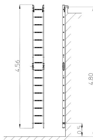
Abb. 31: Einhängeleiter
