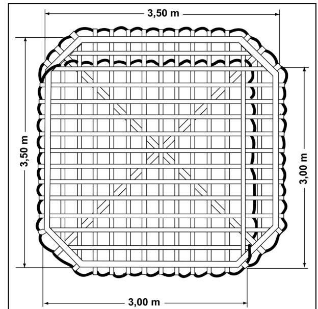
Abb. 19: Sprungtuch ST 8
