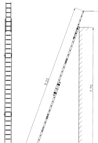
Abb. 30: Anlegeleiter 5-teilig
