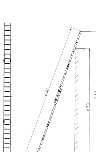
Abb. 29: Anlegeleiter 4-teilig
