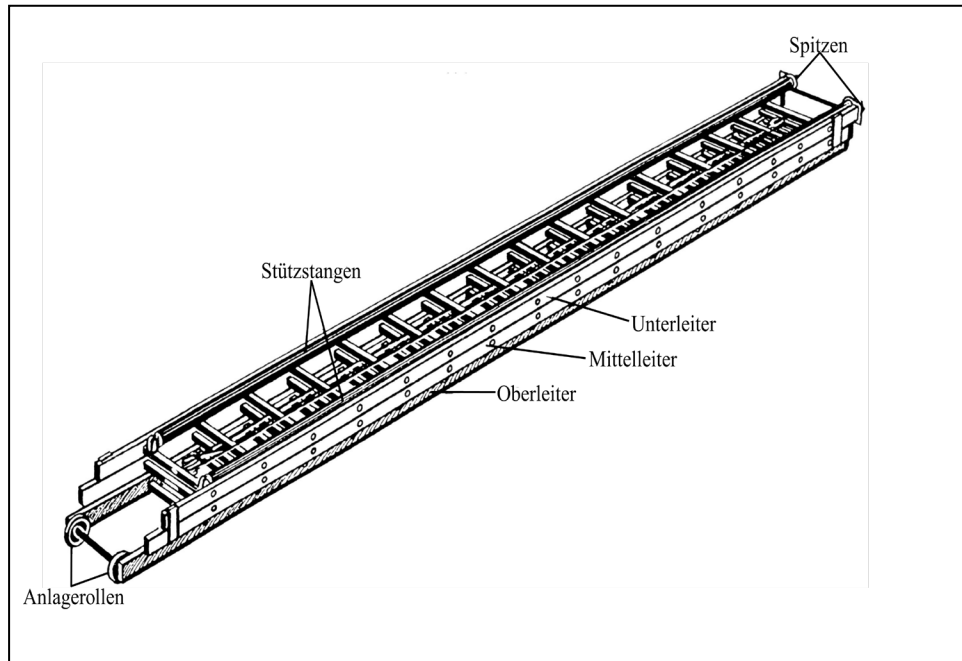
Abb. 8: Dreiteilige Schiebleiter
