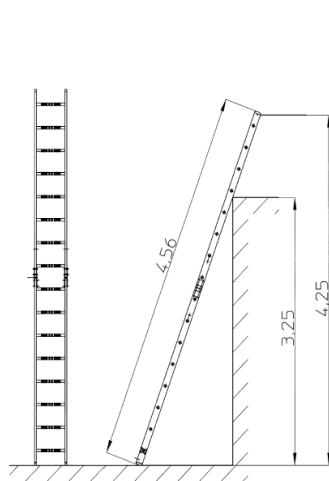
Abb. 27: Anlegeleiter 2-teilig
