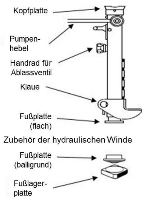
Abb. 30: Hydraulische Winde
