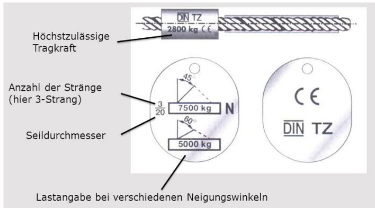
Abb. 17: Kennzeichnung eines Stahldrahtseiles
