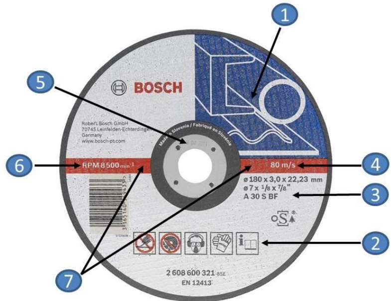
Abb. 37: Trennscheibe
