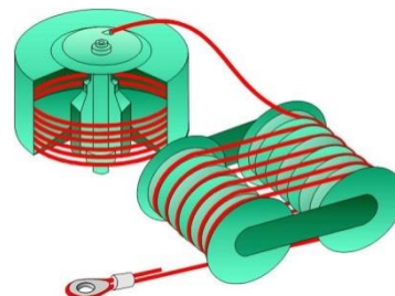
Abb. 23: Treibscheibenwinde
