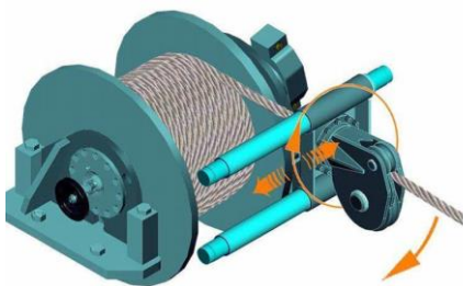
Abb. 22: Trommelwinde
