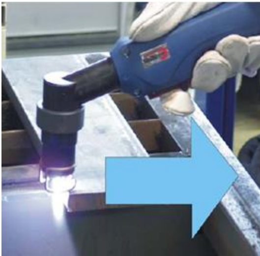
Abb. 46: Beginn am Rand des Werkstückes
