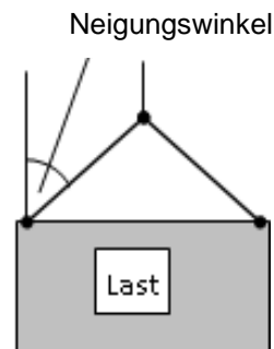
Abb. 15: Neigungswinkel
