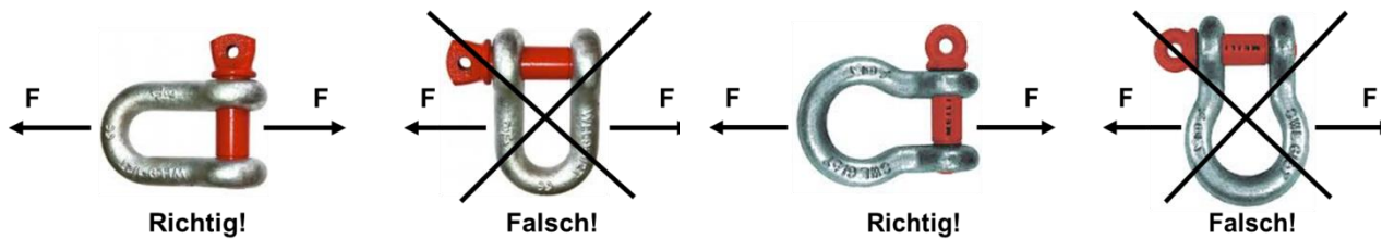
Abb. 19: Zulässige und unzulässige Belastungen am Schäkkel mit gerader und geschweifter Form
