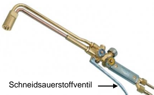
Abb. 44: Schneidbrenner (Griffstück)
