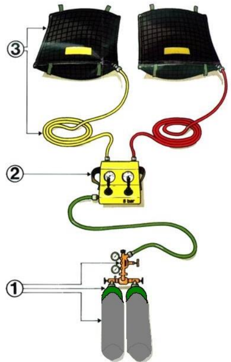
Abb. 27: Hebekissensystem < 1 bar
