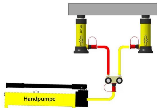
Abb. 33: Mögliche Anordnung der Hydraulikzylinder
