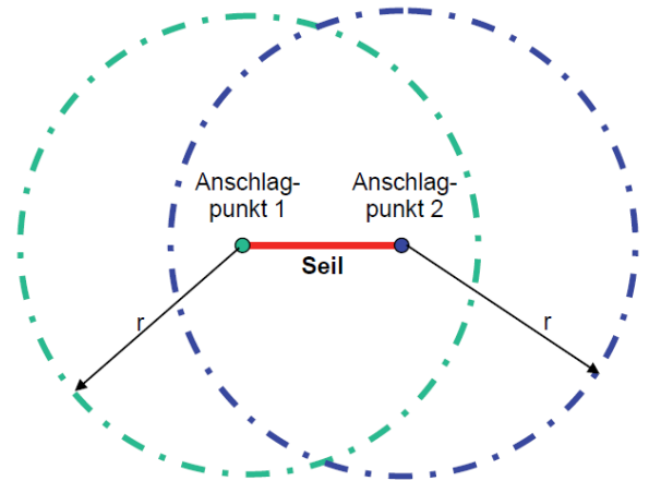
Abb. 21: Sicherheitsabstand
