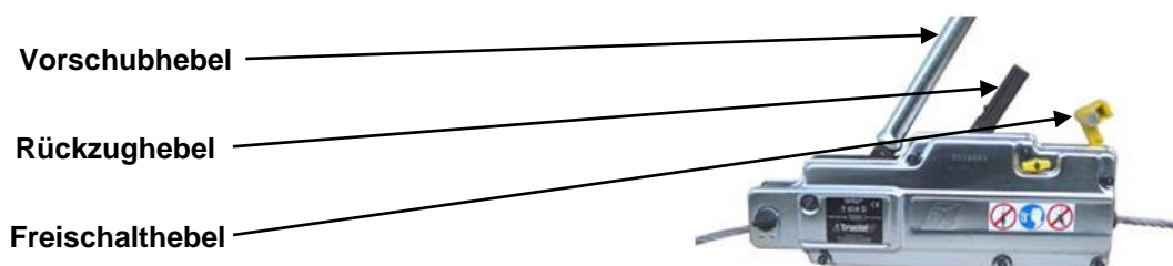
Abb. 20: Mehrzweckzug
