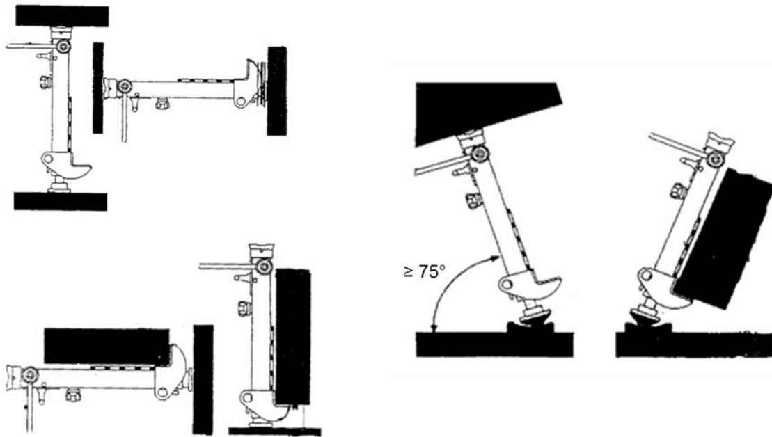
Abb. 31: Einsatzmöglichkeiten der hydraulischen Winde
